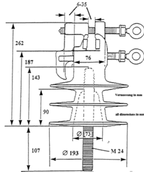
Kabelführung seitlich Cable at the side
