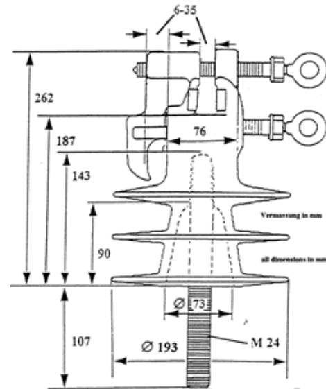
Kabelführung seitlich Cable at the side
